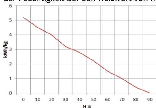
Beziehung zwischen Feuchtigkeit und Heizwert von Holz
