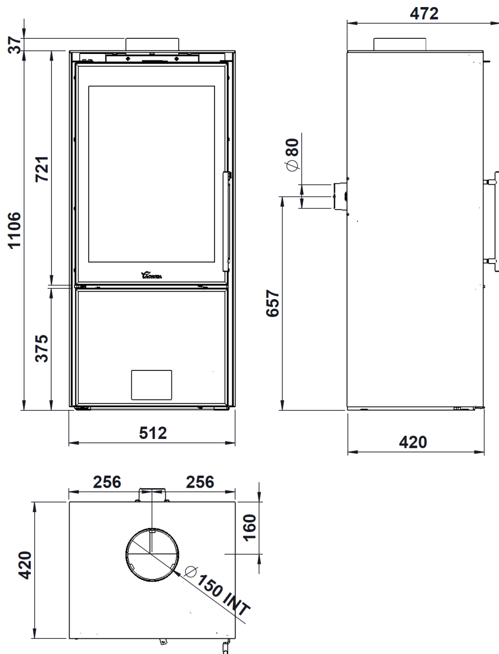
Abmessungen des Geräts in mm CALAIS
