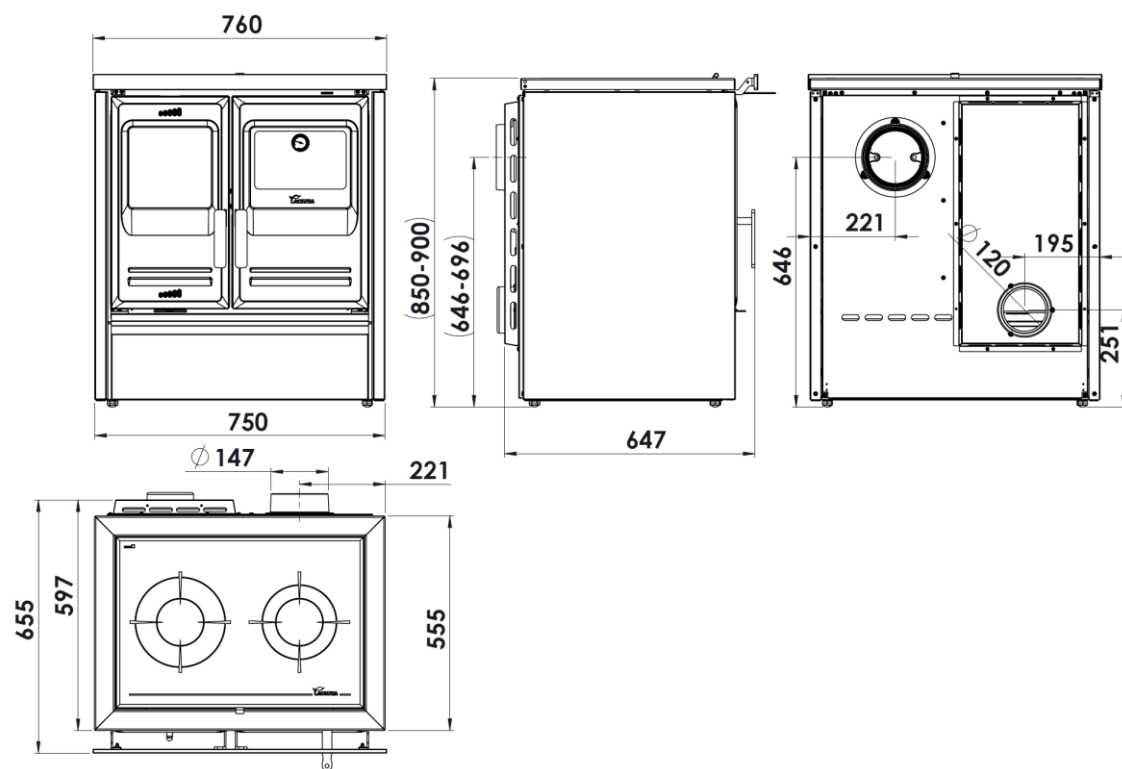
Abbildung Nr. 2 - Abmessungen des Geräts in mm ETNA 5T TOP
