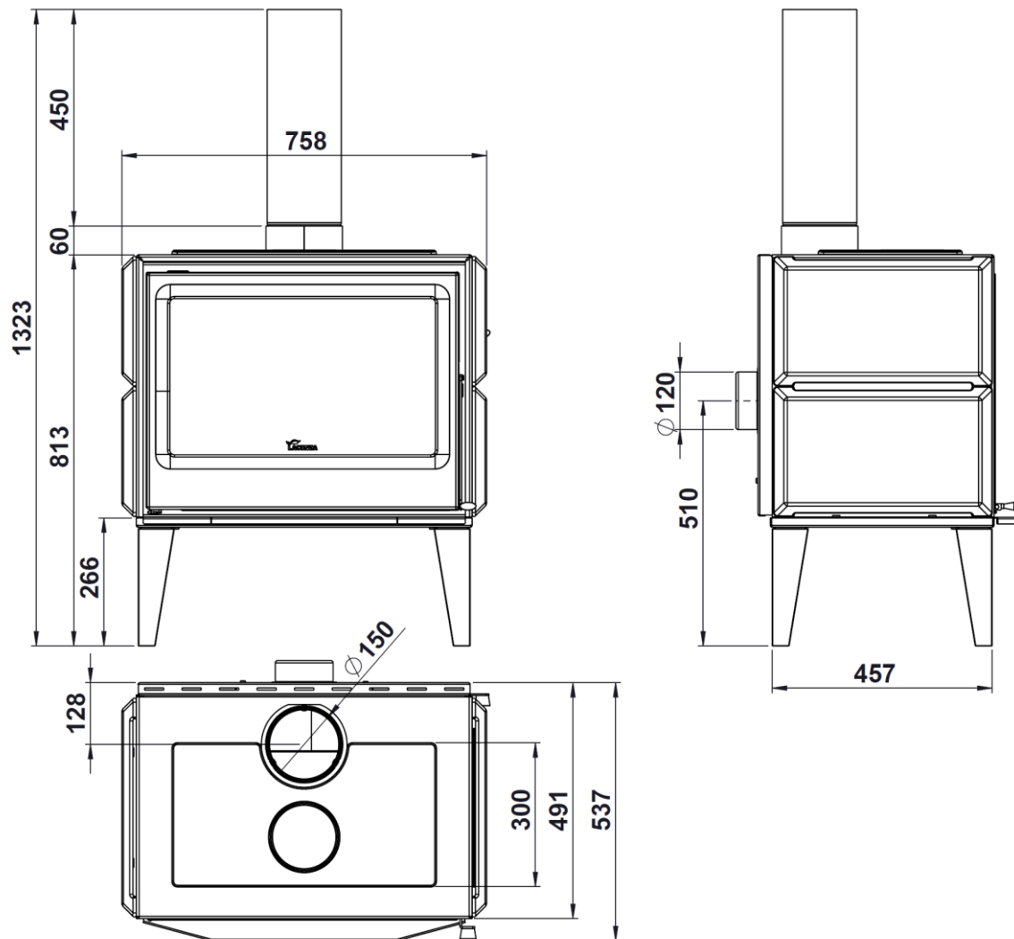
Abbildung Nr.1 - Abmessungen des Geräts in mm MAULE
