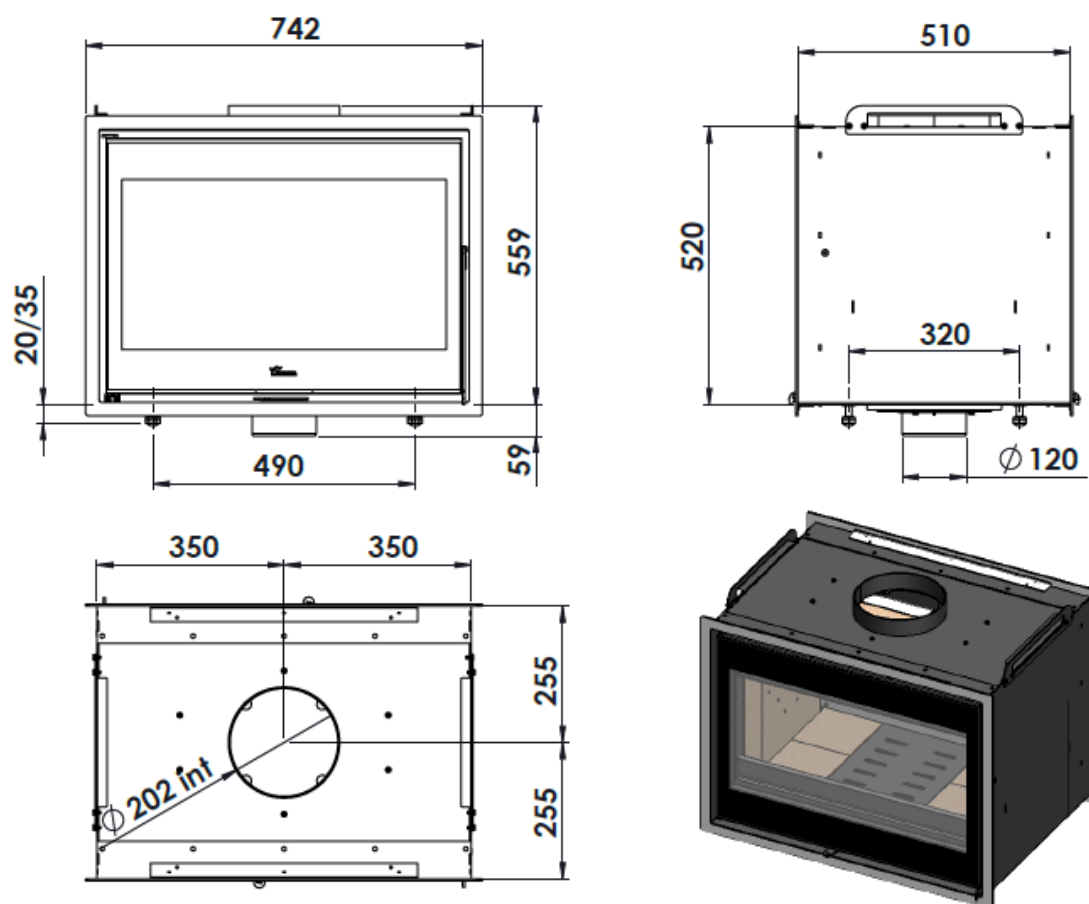
Figura n°1 - Abmessungen in mm del Produkts NICKEL 700
