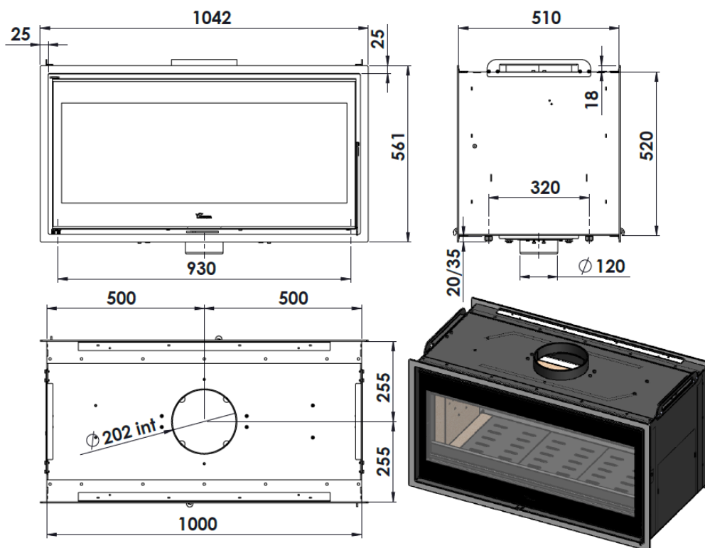
Figura n°3 - Abmessungen in mm del Produkts NICKEL 1000
