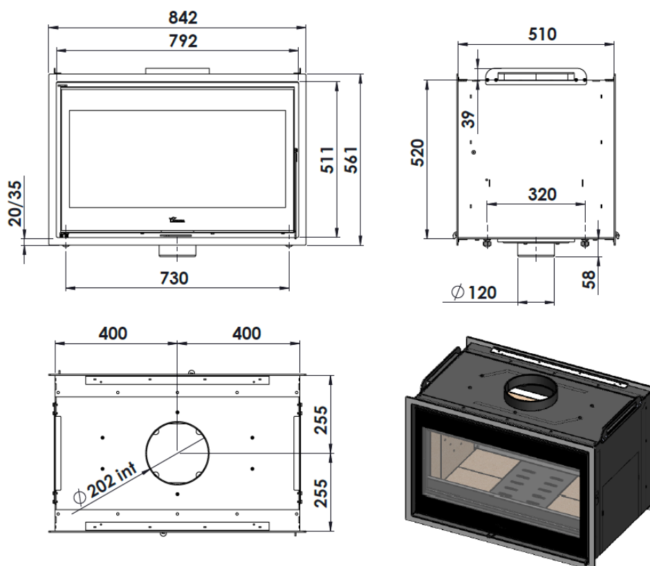
Figura n°2 - Abmessungen in mm del Produkts NICKEL 800
