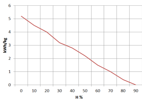
Figura nº5 - Relación entre humedad y poder calorífico de la leña.
