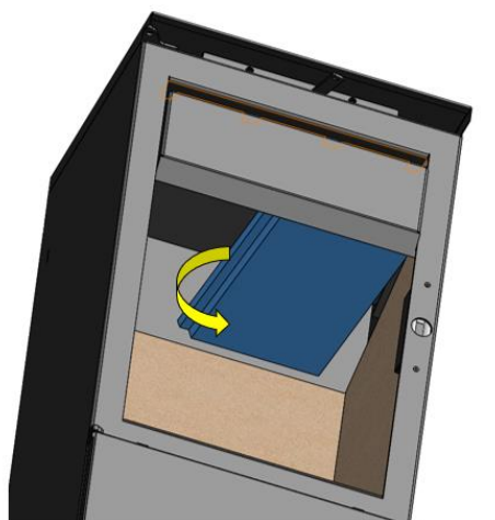
Figura nº7 - Desmontaje de los deflectores inferiores de vermiculita.
