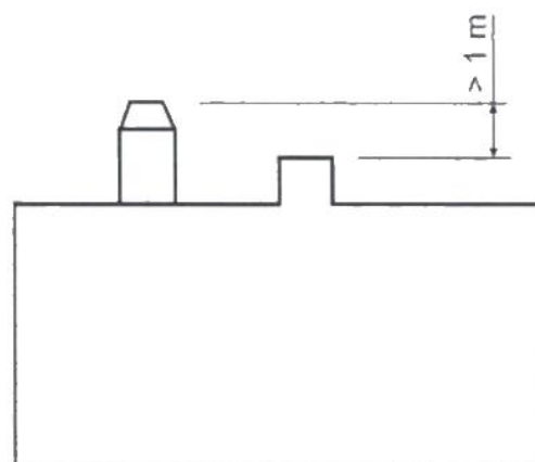
Figura nº2 - Distancias desde el remate hasta la cumbrera del tejado
