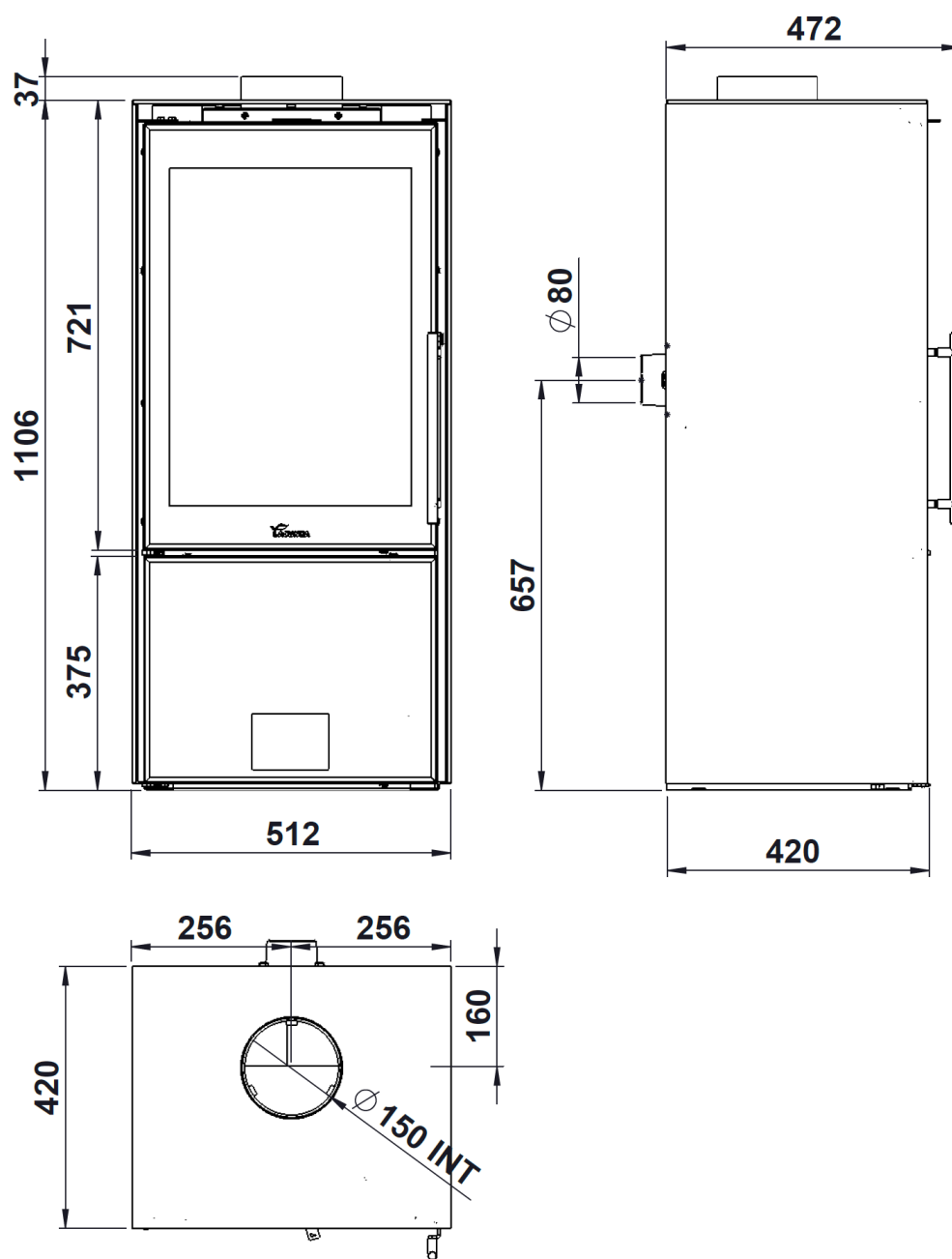
Figura nº2 - Dimensiones en mm del aparato Calais.
