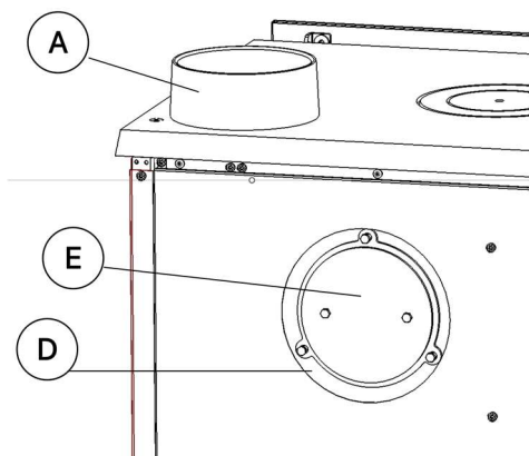
Figura nº7 - Situación final, apta para salida de humos superior.
