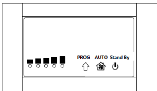
Figura n°46 - Display regulador de aire automático/progresivo Itaca eco
