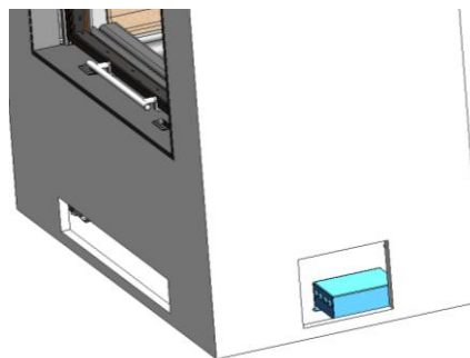
Figura n°20 - Posicionamiento del módulo de potencia frente a la rejilla de ventilación lateral
