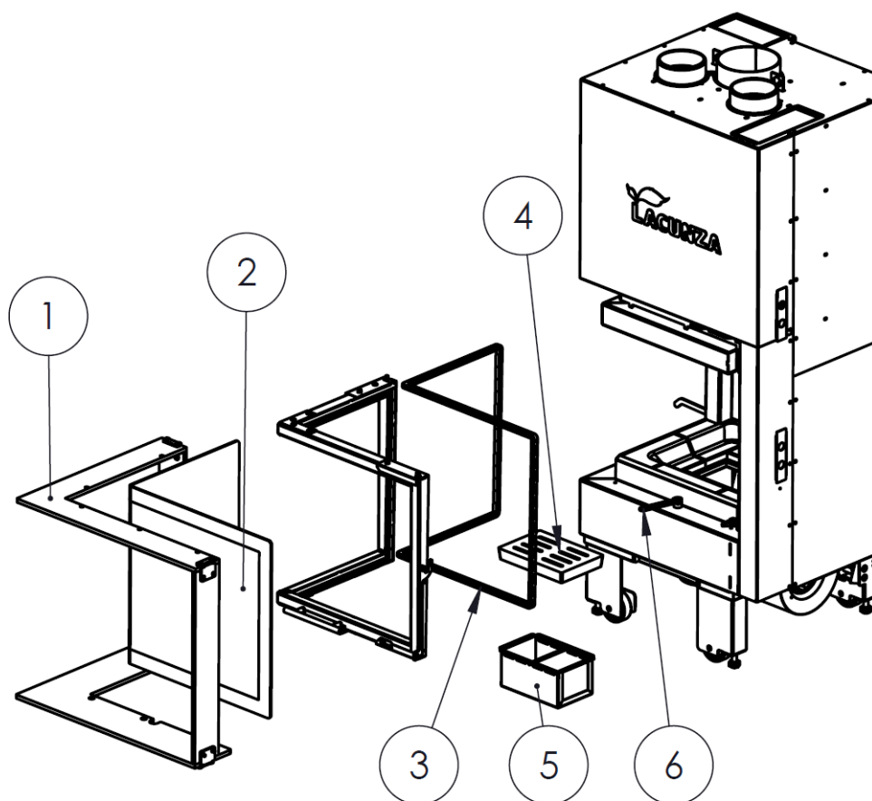
Figura n°46 - Despiece Izaro 60 CLI
