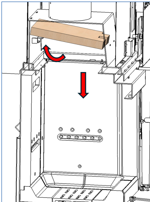
Figura n°35 - Desmontaje del deflector superior Izaro 60 CLI
