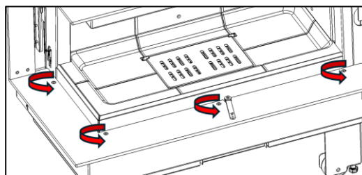
Figura nº15 - Desatornillar los 8 tornillos, 4 superiores y 4 inferiores que amarran el marco exterior
