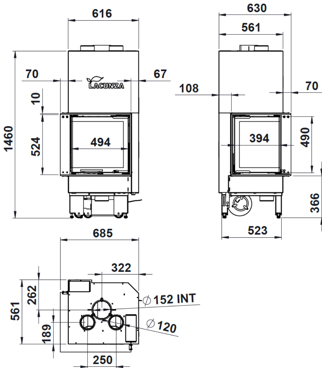
Figura n°1 - Dimensiones en mm del aparato IZARO 60/STAR CLI
