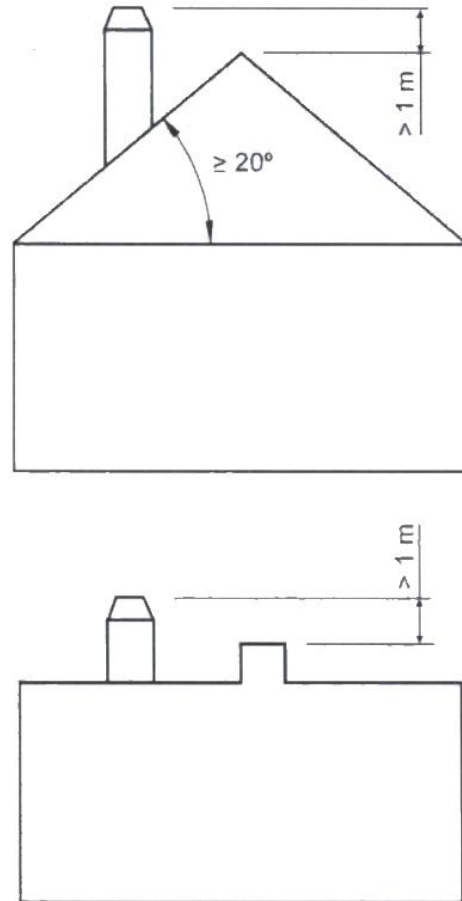
Figura nº25 - Distancias desde el remate hasta la cumbre del tejado
