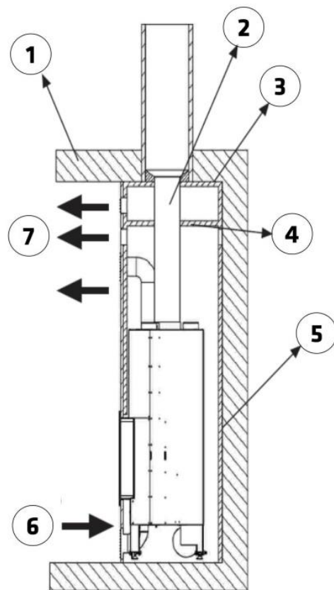
Figura nº9 - Esquema interior del cerramiento
