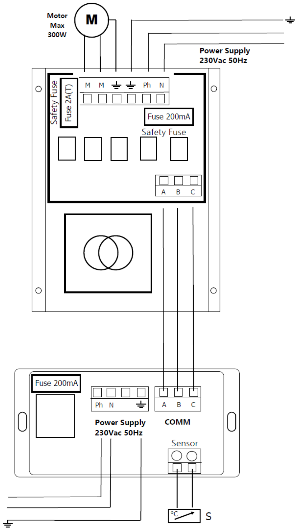
Figura n°20 - Conexiones a realizar en controlador y el módulo de potencia de la Iزارo C/V
