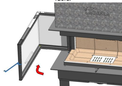
Figura nº43 - Puerta abierta horizontalmente
