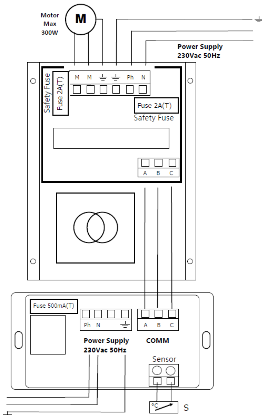
Figura n°20 - Conexiones a realizar en controlador y el módulo de potencia de la Iزارو C/V
