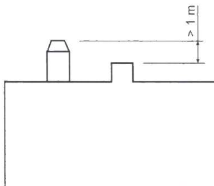
Figura nº15 - Distancias desde el remate hasta la cumbrera del tejado
