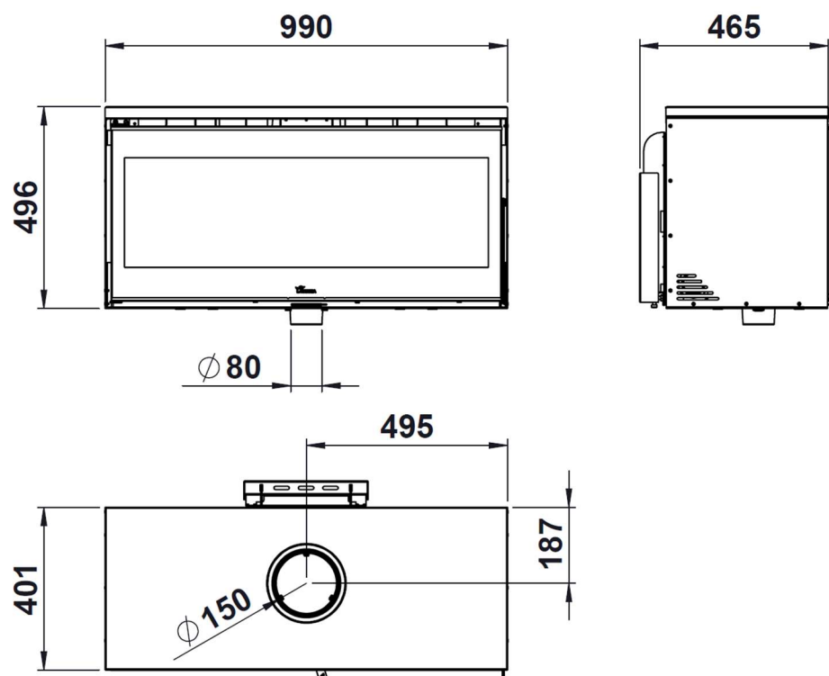
Figura nº10 - Dimensiones en mm del aparato PARIS 1000 MURAL
