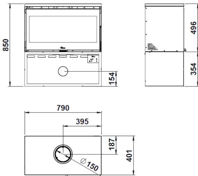
Figura nº5 - Dimensiones en mm del aparato PARIS 800
