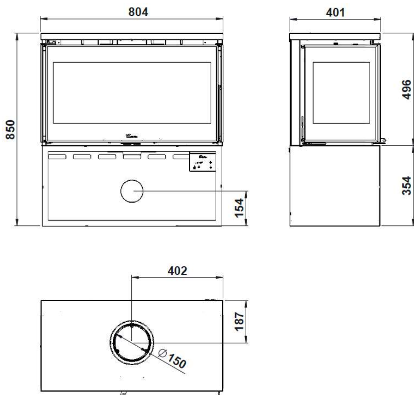
Figura nº6 - Dimensiones en mm del aparato PARIS 800 CLID
