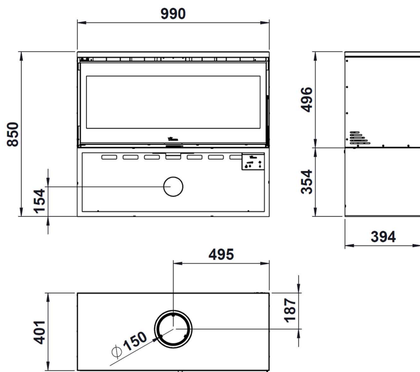
Figura nº9 - Dimensiones en mm del aparato PARIS 1000
