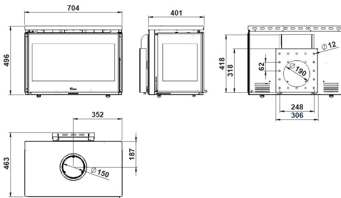
Figura nº4 - Dimensiones en mm del aparato PARIS 700 CLID MURAL
