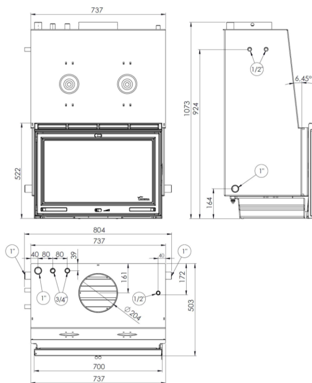
Figura nº3 - Dimensiones en mm del aparato SARRIA 20 - SAKAN 20
