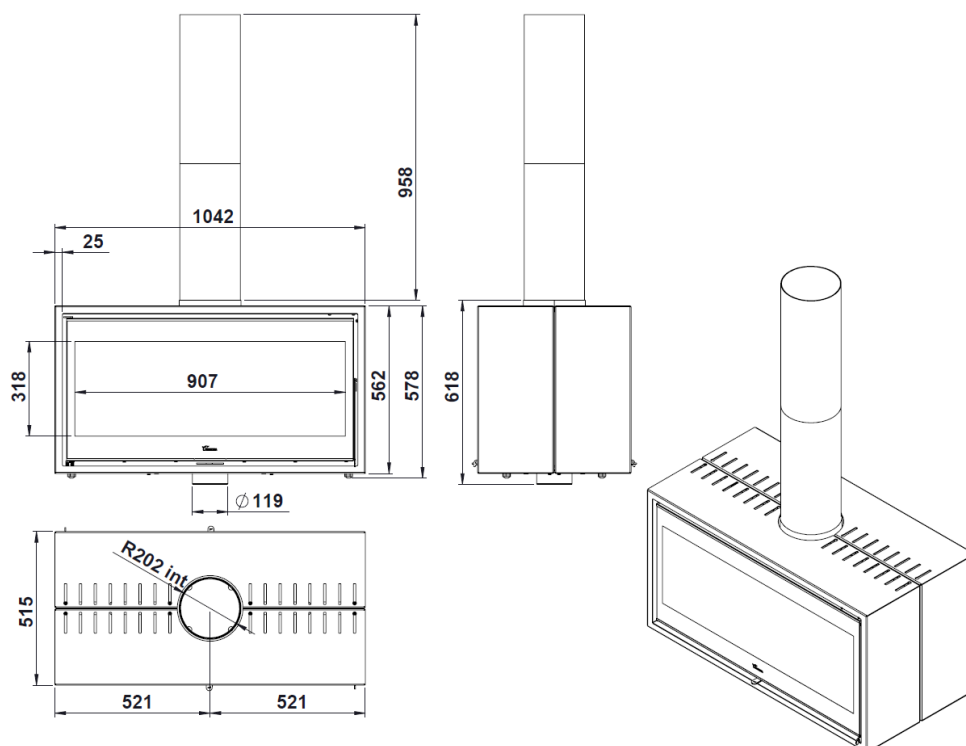
Figura n°3 - Dimensiones en mm del aparato Verona 1000
