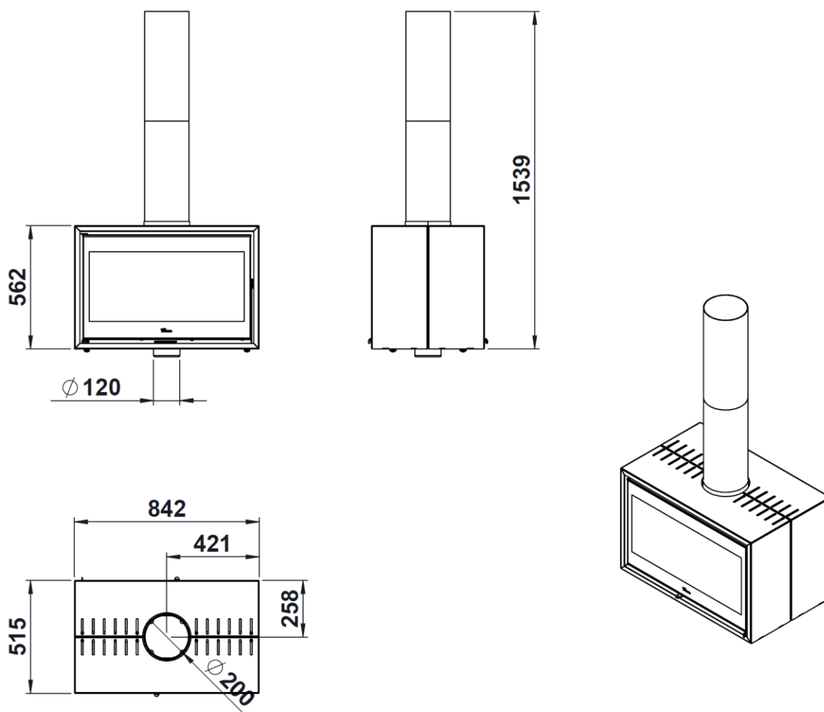
Figura nº1 - Dimensiones en mm del aparato Verona 800
