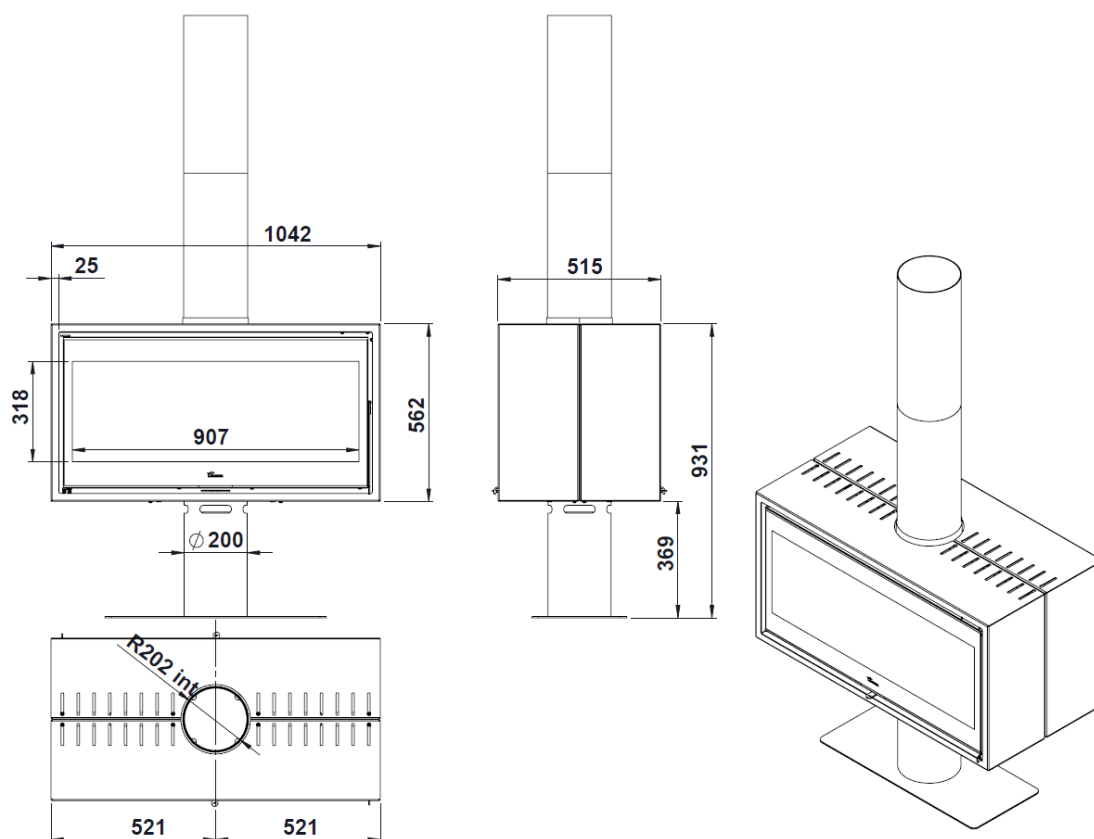
Figura nº4 - Dimensiones en mm del aparato Verona 1001
