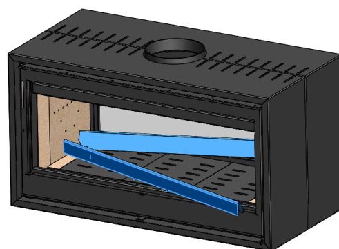
Figura nº19 - Extraemos los dos separadores del hogar
