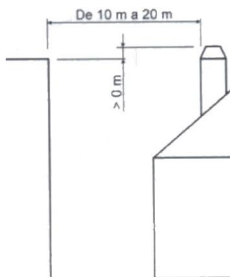
Figura n°16 - Distancias desde el remate hasta objetos entre 10
