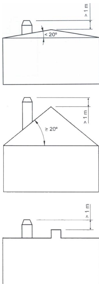
Figura n°4 - Distâncias desde o acabamento até à cumeeira do telhado
