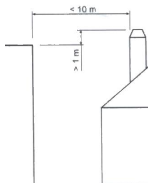
Figura n°5 - Distâncias desde o acabamento até objetos a menos de 10m
