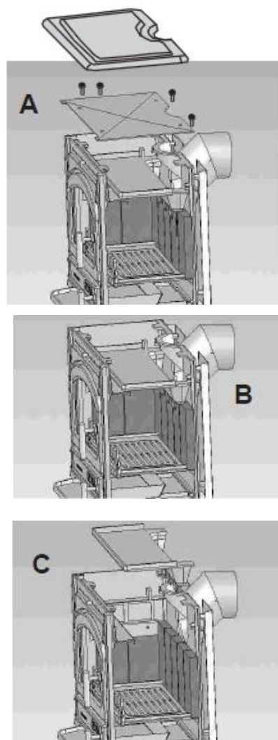
Figura nº9 - Desmontagem do defletor
