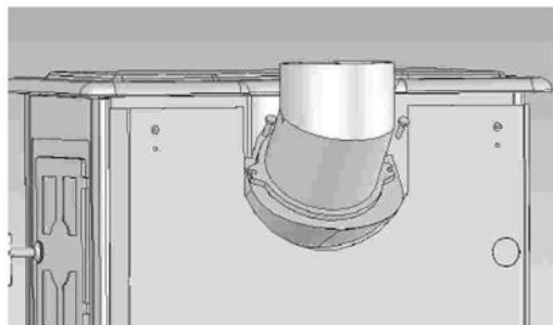
Figura nº3 - Esquema para saída de fumos traseira
