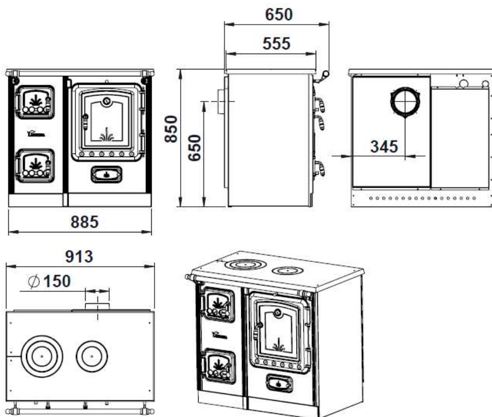
Figura nº2 - Dimensões em mm do aparelho Lís 7T
