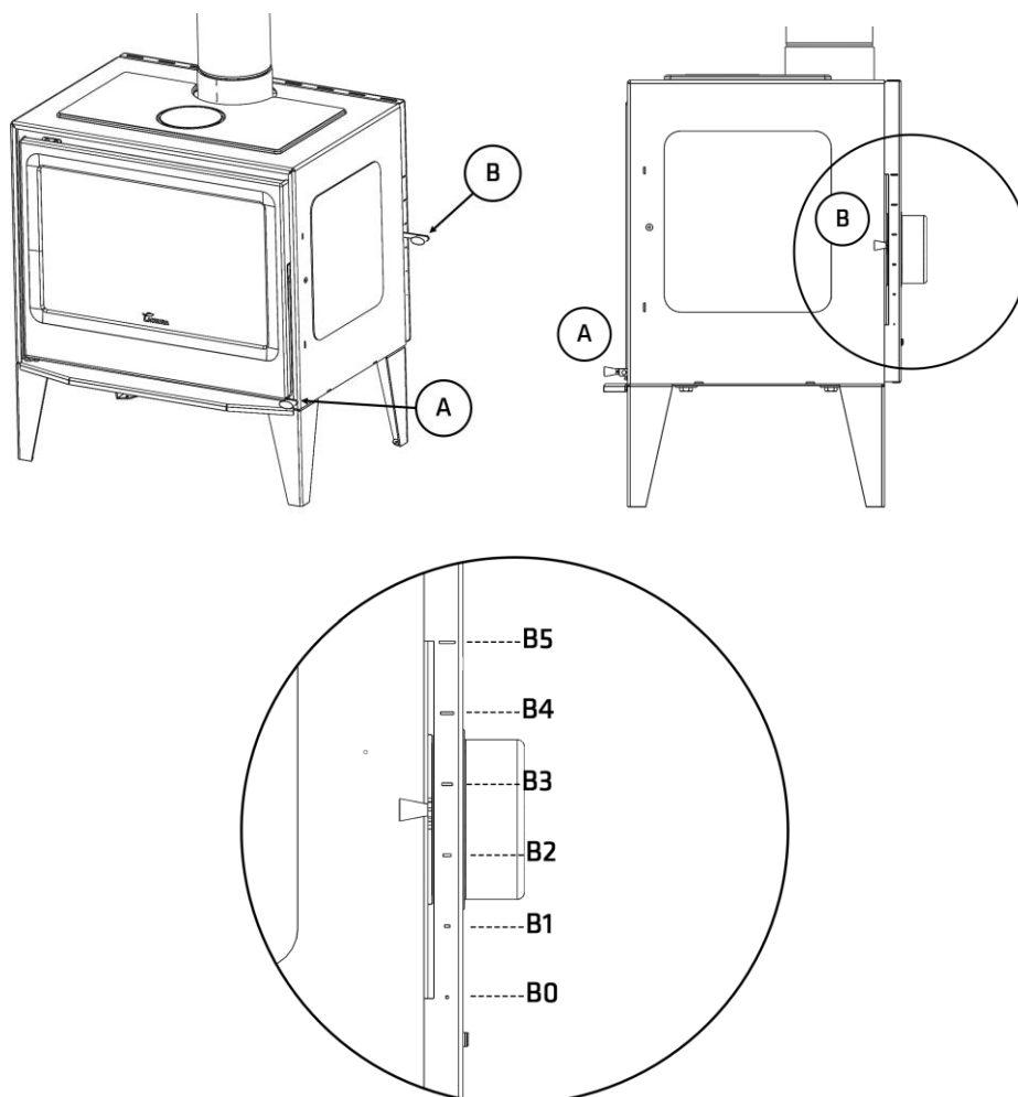
Figura n.º8 - Elementos de funcionamento do aparelho
