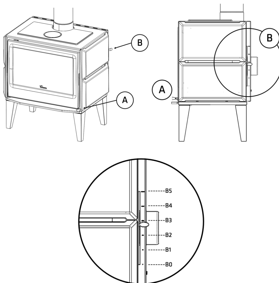
Figura nº8 - Elementos de funcionamento do aparelho
