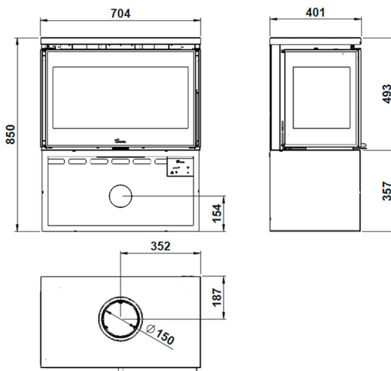
Figura n°2 - Dimensões em mm do aparelho PARIS 700 CLID
