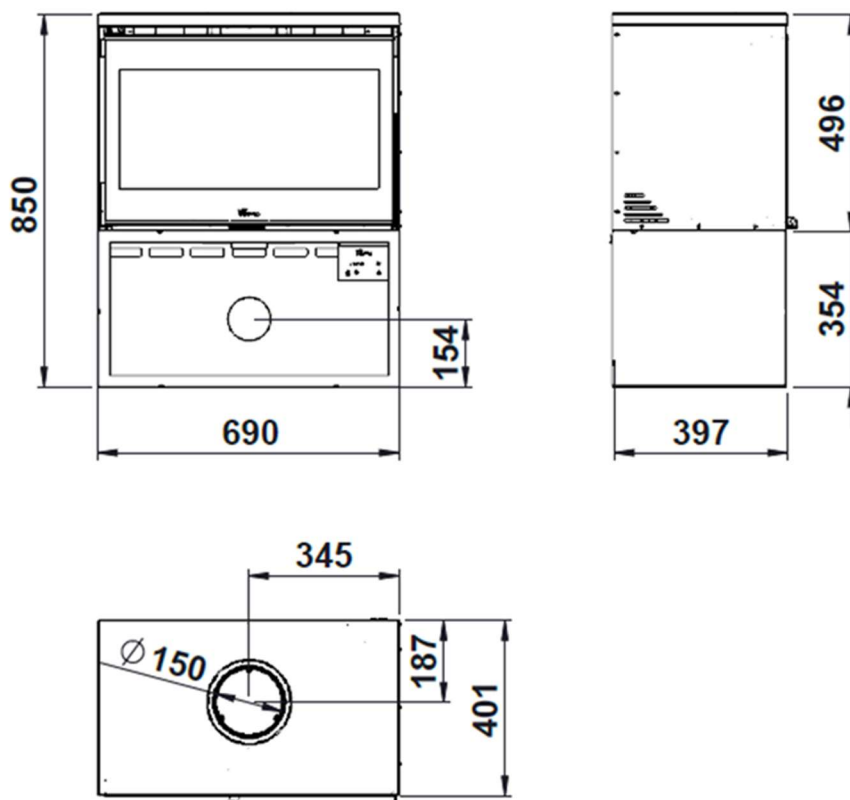
Figura n°1 - Dimensões em mm do aparelho PARIS 700
