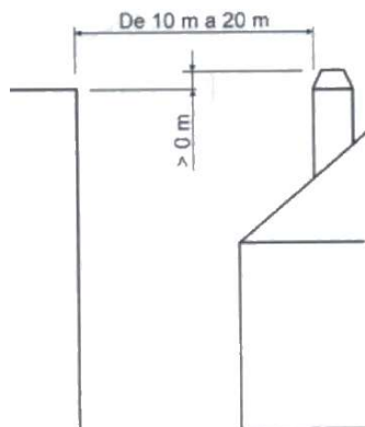
Figura n°5 - Distanza tra la finitura e oggetti tra 10 e 20 m
