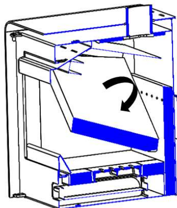
Figura n°10 - Estrazione dei deflettori in vermiculite
