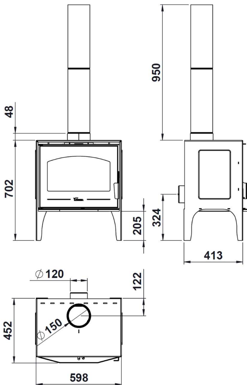
Figura n°1 - Dimensioni in mm dell'apparecchio serie CALPE
