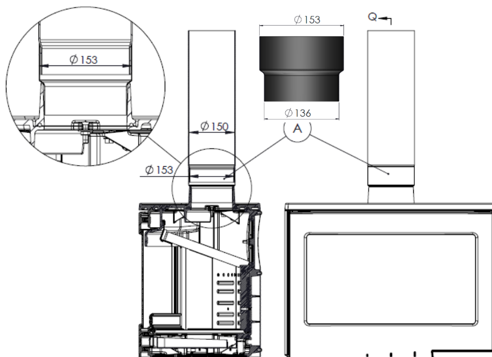
Figura nº4 - Collegamento allo scarico fumi con adattatore (A) in dotazione
