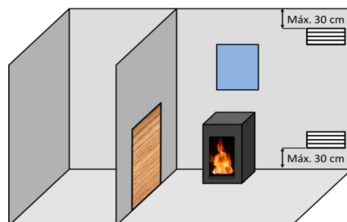
Figura nº5 - Schema orientativo per griglie di ventilazione
