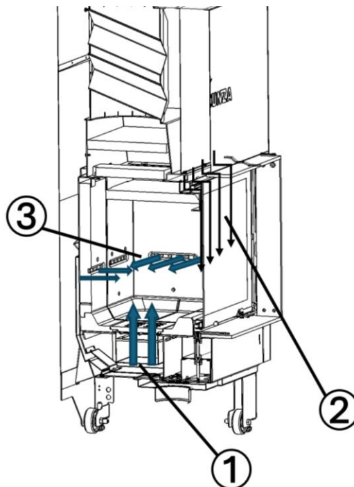
Figura n°28 - Ingresso d'aria combustione
