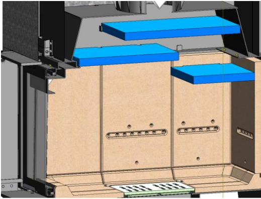
Figura n°34 - Vista in sezione dell'Izaro 100 CLI con i 3 deflettori posizionati
