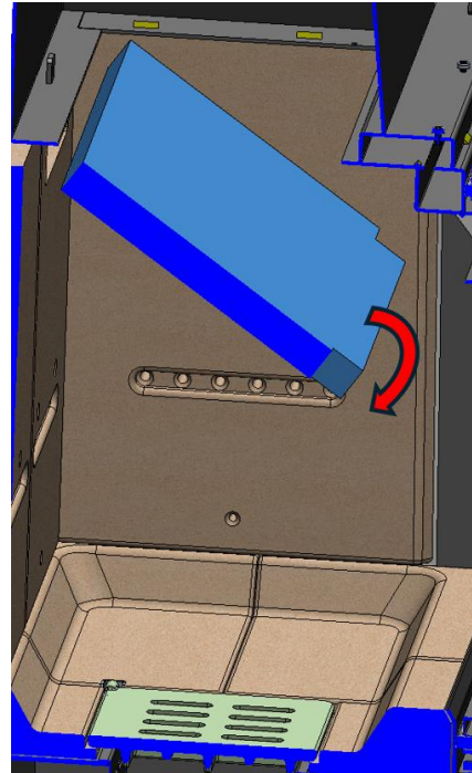
Figura n°37 - Smontaggio del deflettore superiore dell'Iزارo 100 CLI
