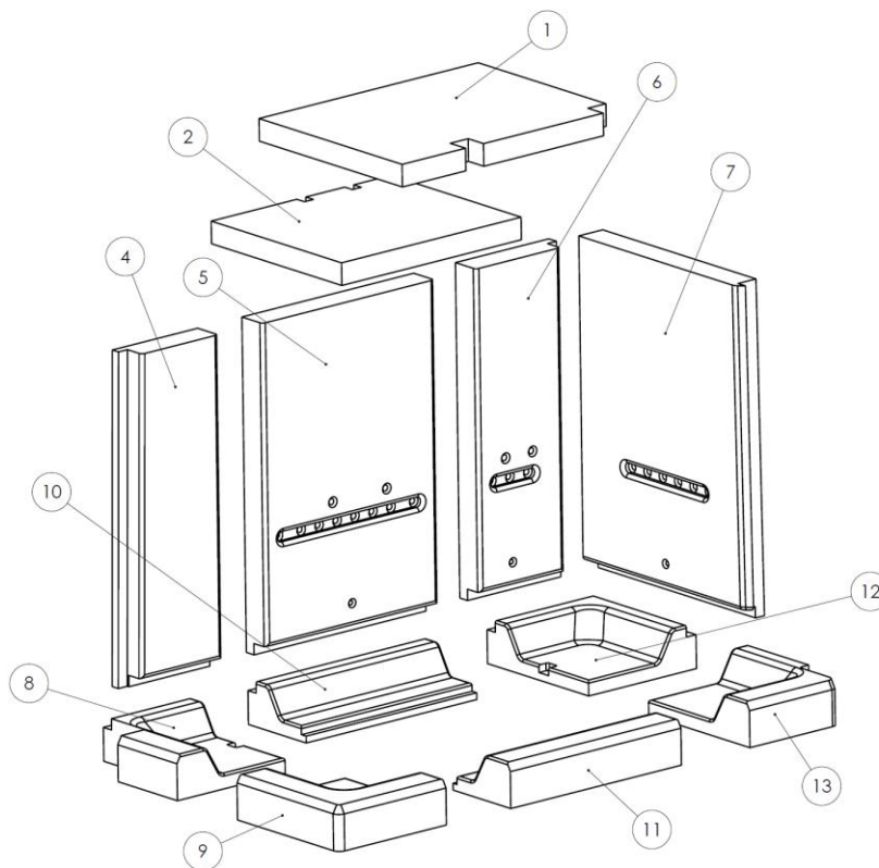
Figura nº49 - Vista esplosa vermiculite IZARO 80 CLI
