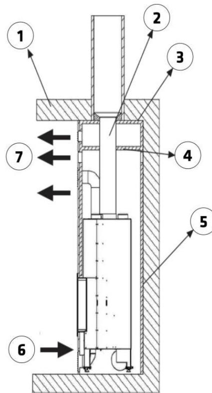
Figura n°9 - Schema interno del rivestimento
