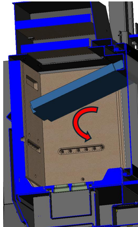
Figura n°35 - Smontaggio del deflettore inferiore dell'Izaro 100 CLI
