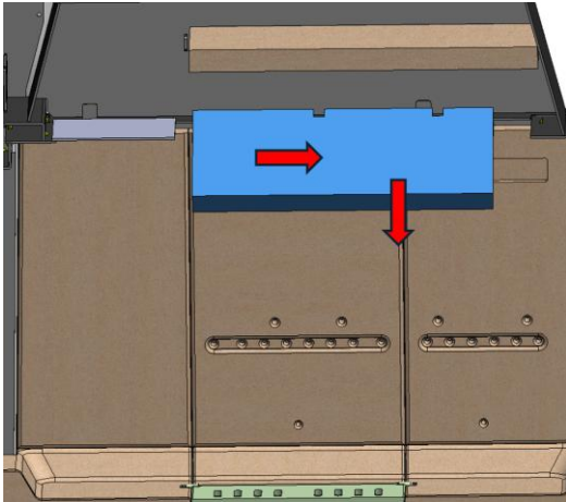
Figura n°36 - Smontaggio del deflettore medio Iزارo 100 CLI
