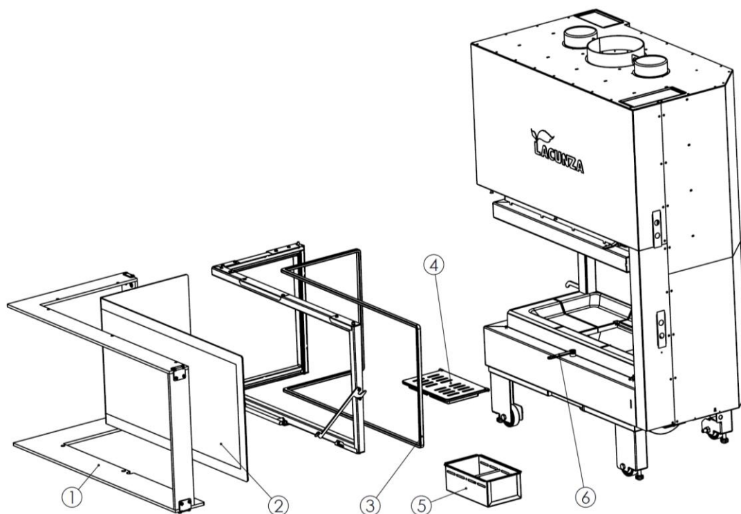
Figura n°48 - Pezzi principali Izaro 80-100 CLI
