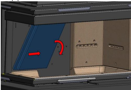
e- Rimuovere la piastra posteriore sinistra (4) spostandola verso l'interno e lasciandola cadere in avanti.
