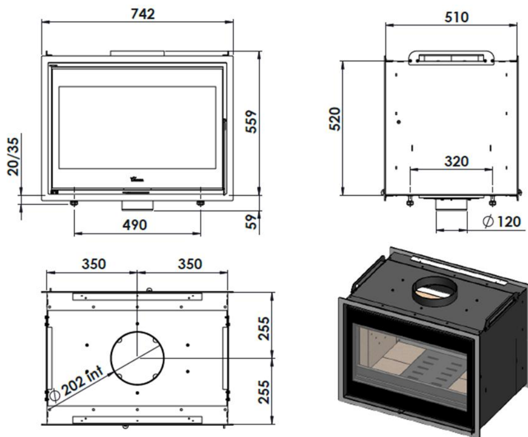
Figura n°1 - Dimensioni in mm dell'apparecchio Nickel 700
