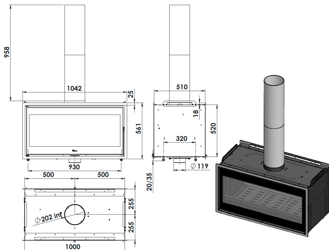
Figura n°3 - Dimensioni in mm dell'apparecchio Nickel 1000
