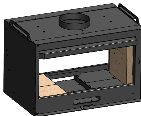
Figura n°19 - Estraiamo i refrattari situati davanti e dietro la griglia in ghisa
