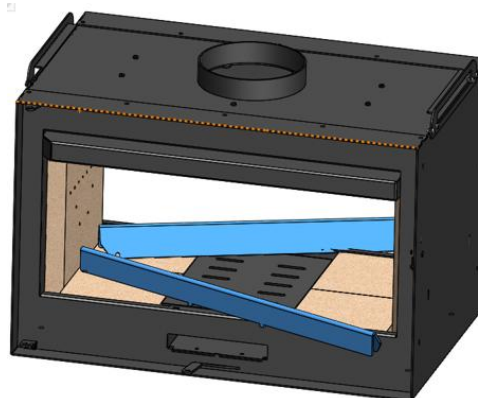
Figura n°17 - Estraiamo i due separatori del focolare
