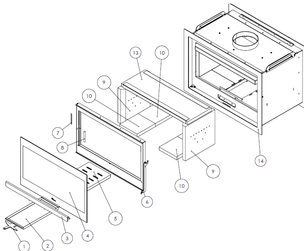
Figura n°23 - Pezzi principali Nickel 700/800/1000
