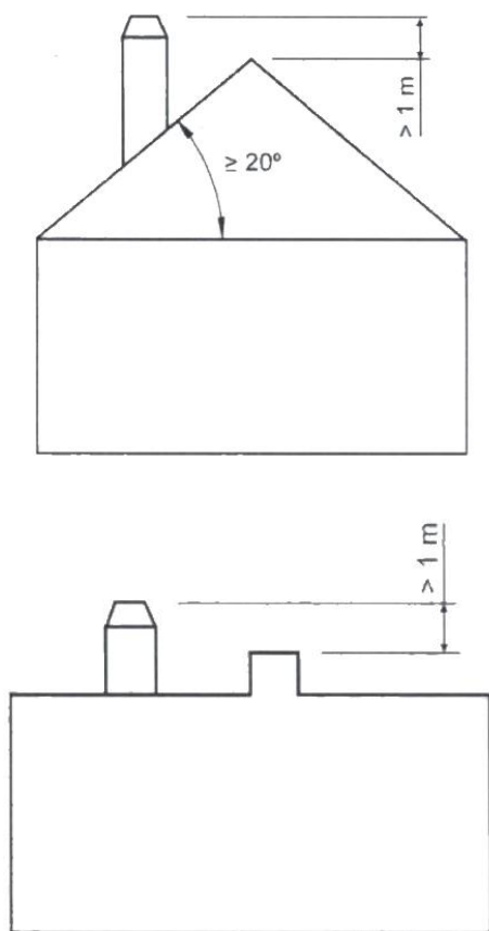
Figura n°12 - Distanza tra la finitura e il colmo del tetto
