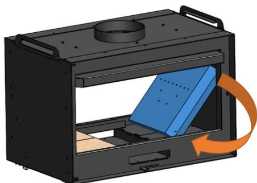
Figura n°20 - Ruotare il lato refrattario in modo che il deflettore possa cadere.
