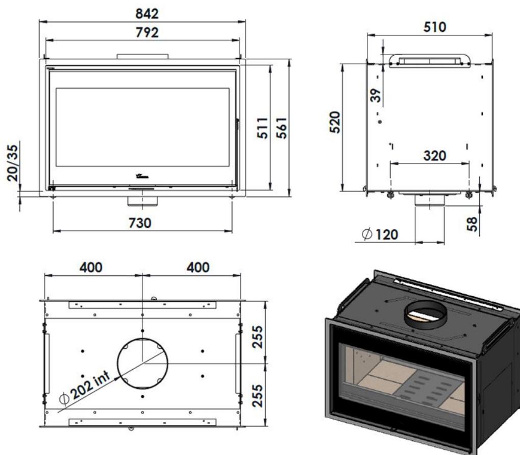
Figura n°2 - Dimensioni in mm dell'apparecchio Nickel 800
