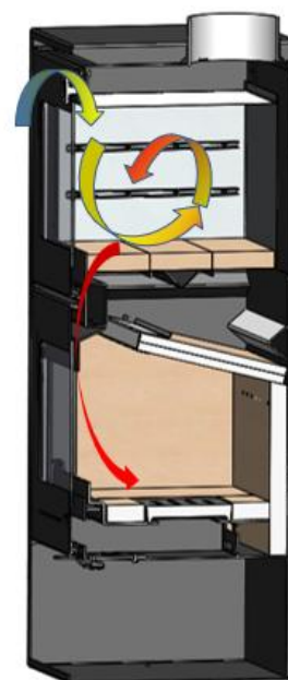
Figura n°9 - Schema sistema di estrazione di vapore
