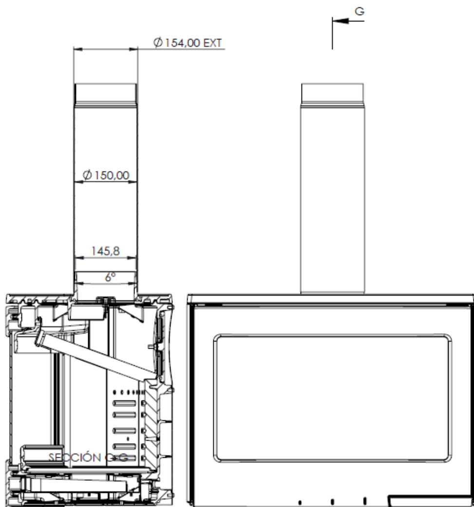
Figura nº2 - Collegamento allo scarico fumi senza l'adattatore in dotazione
