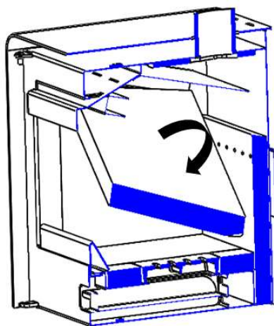
Figure n°11 - Extraction des déflecteurs en vermiculite
