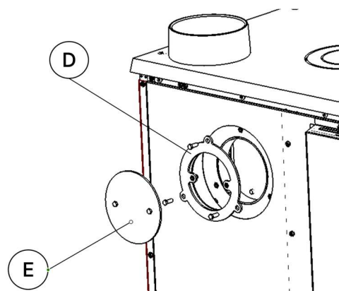
Figure n°6 - Nous plaçons l'adaptateur et le couvercle
