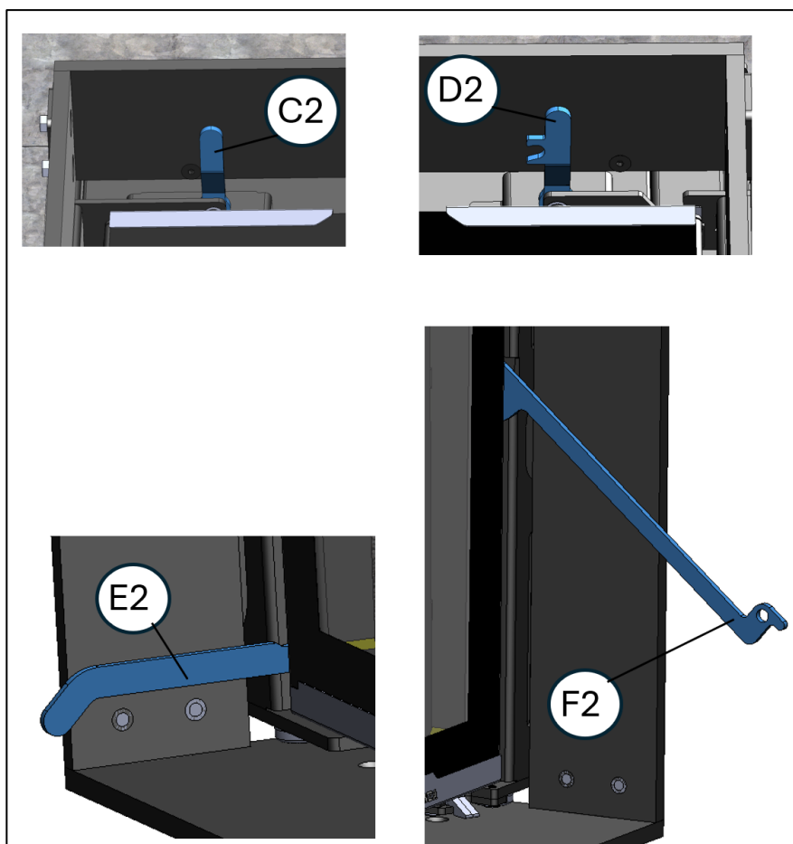
Figure n°29 - Éléments de fonctionnement de l'appareil IZARO 80-100 CLI
