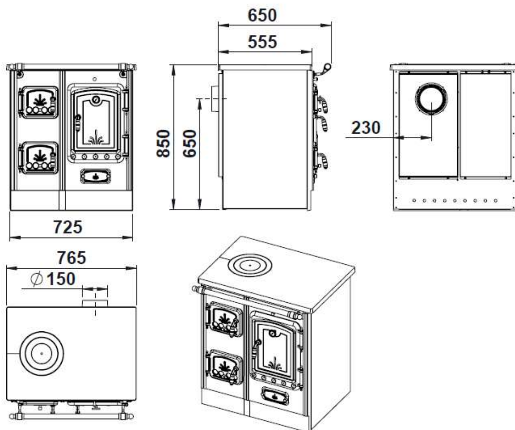
Figure n°1 - Dimensions en mm de l'appareil Lis 5T
